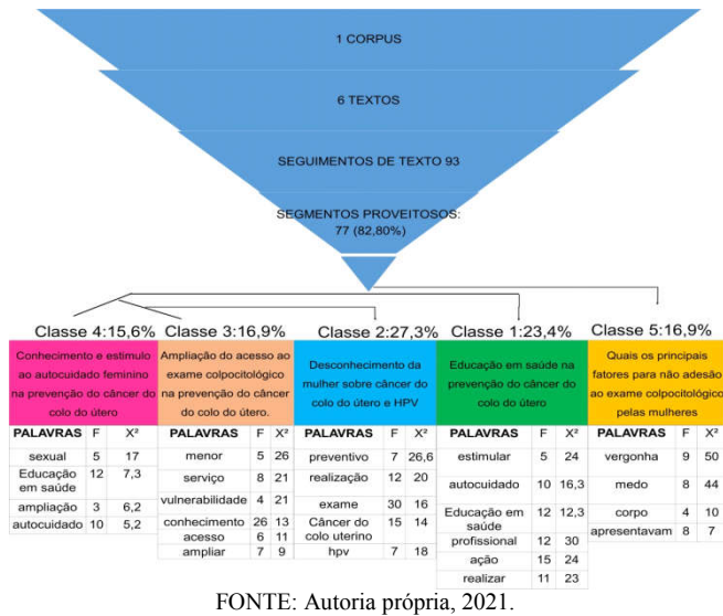
Figura 2. Dendrograma de Classificação Hierárquica Descendente (CHD)
